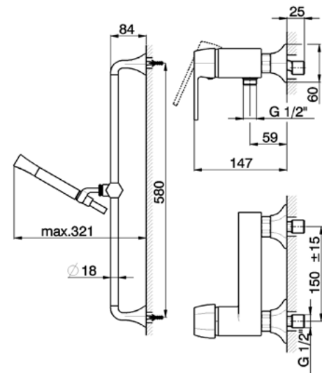
CH000464 Completo Monocomando Doccia Shower Mixer Set Ensemble Mitigeur Douche
