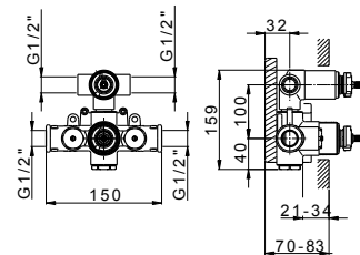
ZA019100 Parte Incasso Termostatico 2 Uscite 2-Outlet Thermo Concealed Part Partie Encastrée Thermo 2 Sorties
