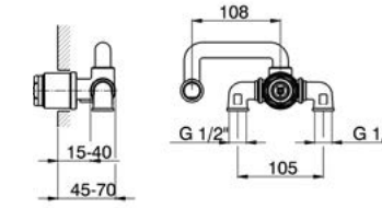
ZA006510 Parte Incasso Monocomando Lavabo Basin Mixer Concealed Part Partie Encastrée Mitigeur Lavabo
