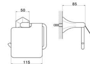
CE090420 Porta Rotolo Roll Holder Porte-Papier
