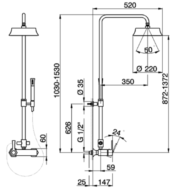
CH004024 CombiDoccia Monocomando CombiShower Mixer CombiDouche Mitigeur
