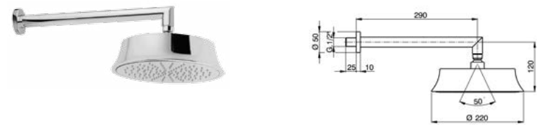
DS013590 Braccio e Soffione Doccia Shower Arm & Head Bras et Tête de Douche
