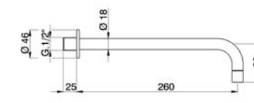
ZA002251 Bocca di Erogazione Filler Spout Bec Verseur
