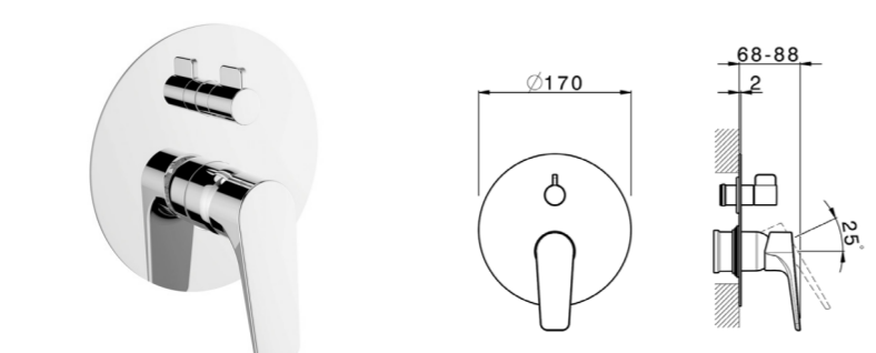
RK 002300 Parte Esterna Monocomando Vasca/Doccia Bath/Shower Mixer Exposed Part Partie Décor Mitigeur Bain/Douche per/for /pour EASY Box
