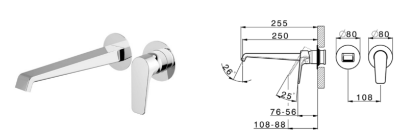
RL 005511 Parte Esterna Monocomando Lavabo Basin Mixer Exposed Part Partie Apparente Mitigeur Lavabo per/for /pour EASY Box
