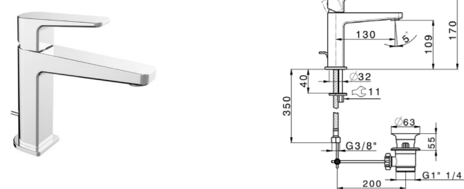
RK 000494 Monocomando Lavabo Basin Mixer Mitigeur Lavabo
