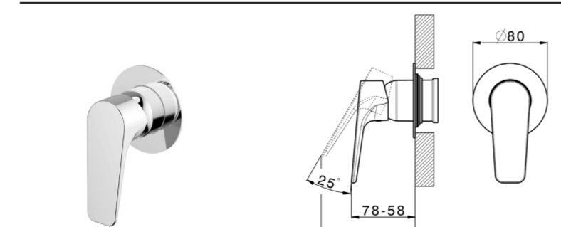
RK 003000 Parte Esterna Monocomando Doccia Shower Mixer Exposed Part Partie Décor Mitigeur Douche per/for /pour ZA 005300 - ZA 005301
