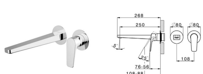
RK 005511 Parte Esterna Monocomando Lavabo Basin Mixer Exposed Part Partie Apparente Mitigeur Lavabo per/for /pour EASY Box
